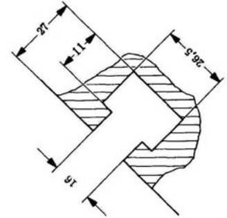
T-Nutenabmessungen am Maschinenbett
